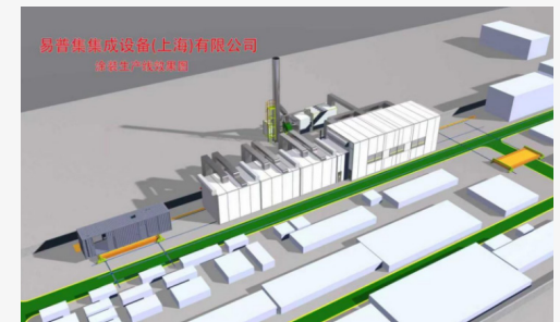
▲ 自動噴塗線廢氣處理系統效果圖
